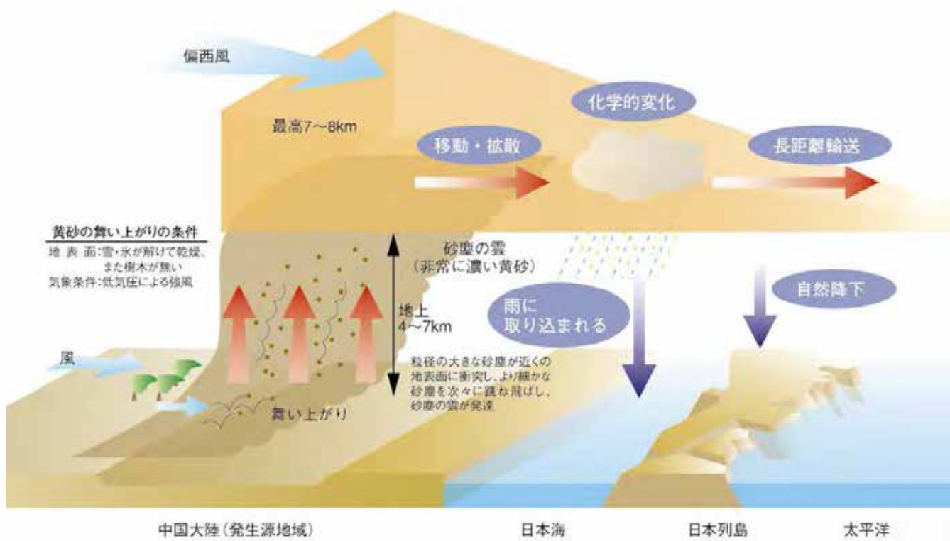
図 1-4 黄砂の発生・輸送機構
