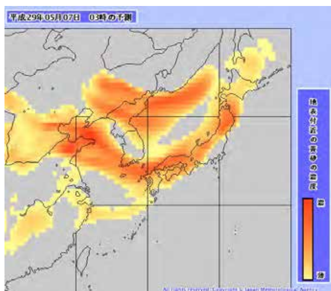
図 4-2 黄砂情報（予測図） (2017 年 5 月 7 日)
