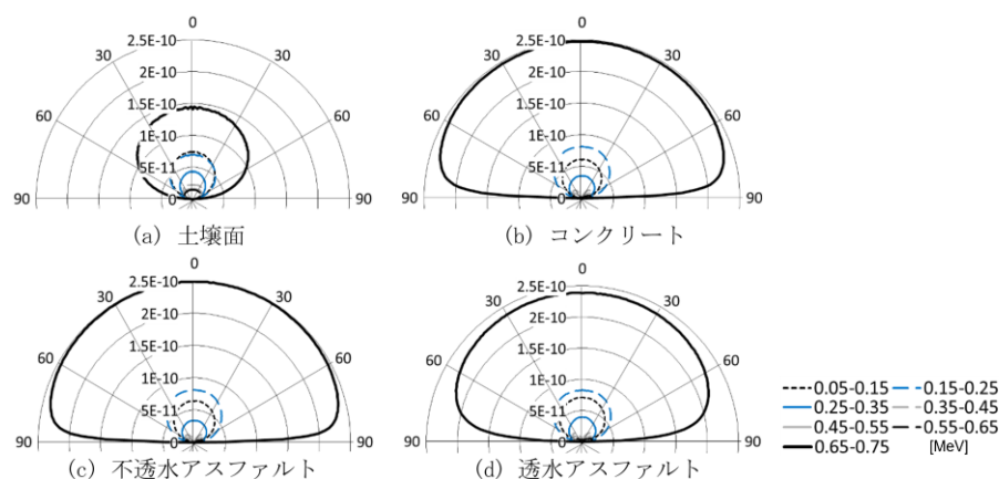
図 10 地表面種別による 1 Bq あたりの \gamma 線射出特性 [Sv/sr]
