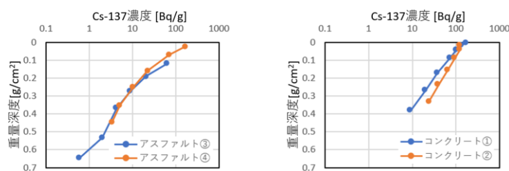
図7 同施設のアスファルト(左)、コンクリート(右)の深度分布
