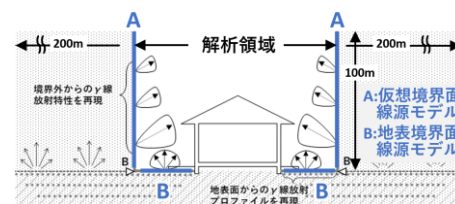
図5 仮想境界面（A、B）
