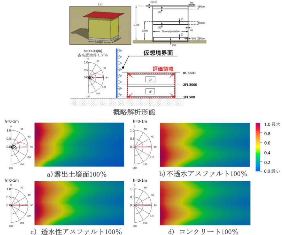
図 13. 境界モデルによる木造2層建物内空間線量率解析
