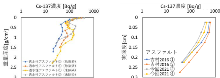
図8 透水性アスファルト
