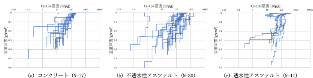
図 11 Cs-137 深度分布調査結果
