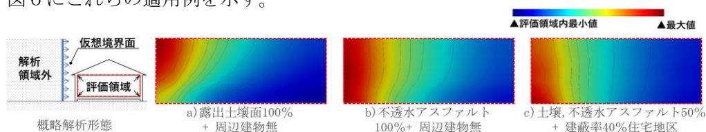
図6 仮想境界モデルによる建物内空間線量率（各最大値で規準化）
