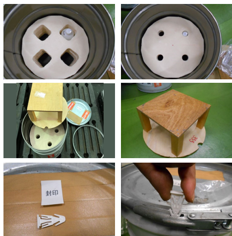
潰れ防止のための中蓋及び封印用鍵
