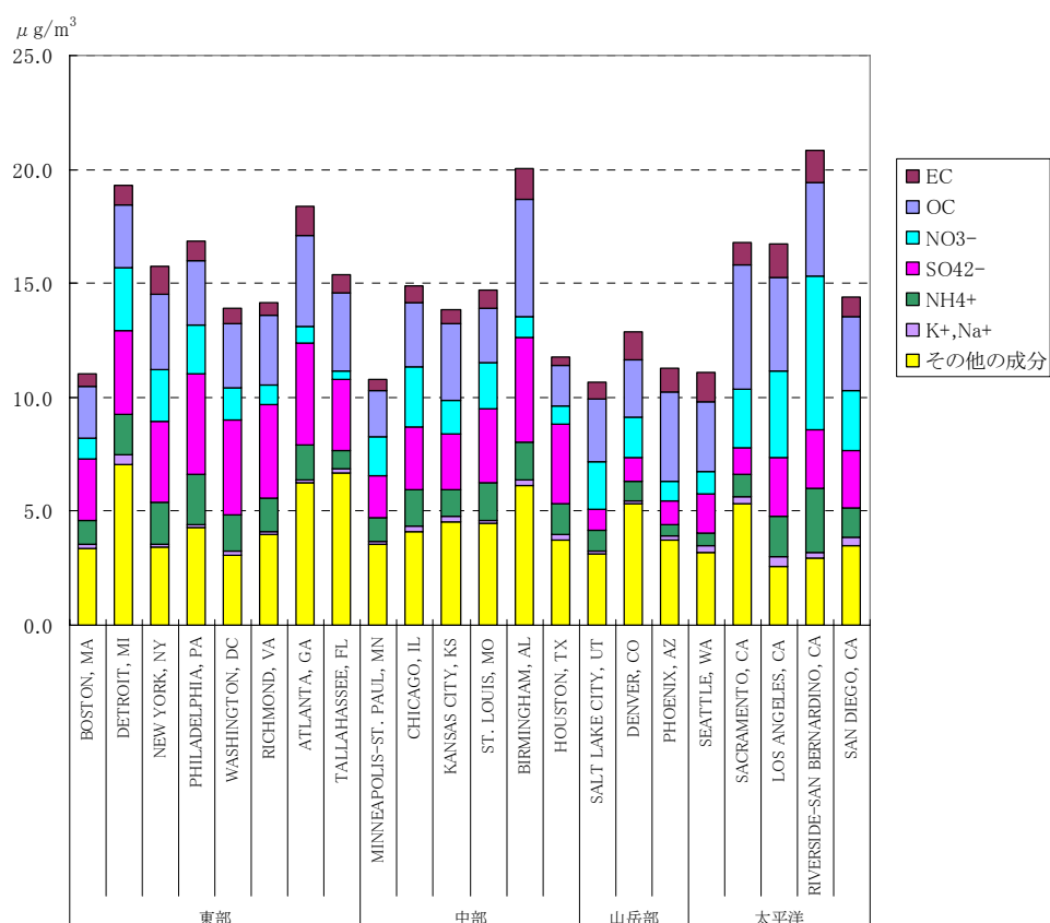
図2 米国の都市におけるPM 2.5 成分データ(2006年度通年)
