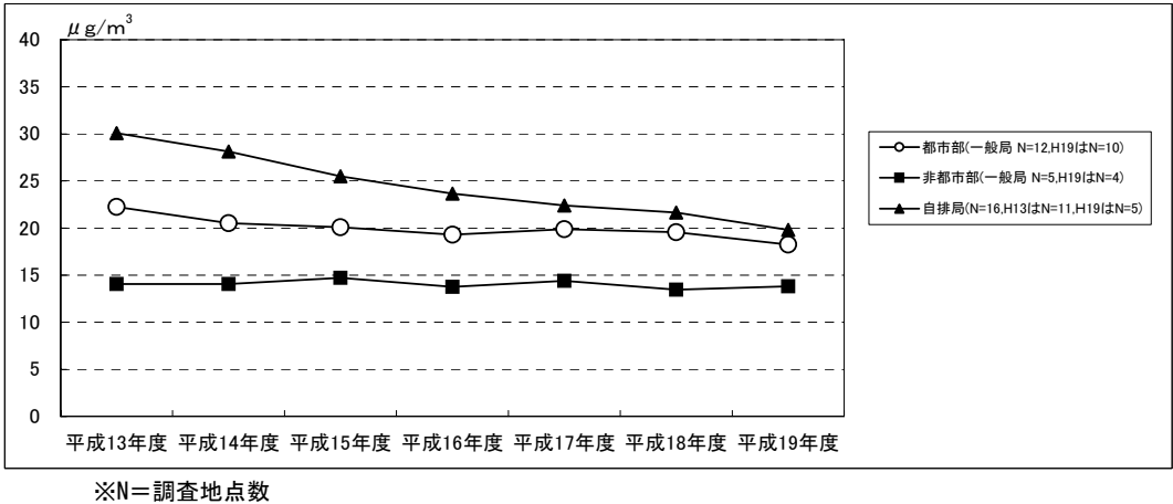
図1 PM 2.5 (50℃加熱方式TEOM)質量濃度の年平均値の経年変化
