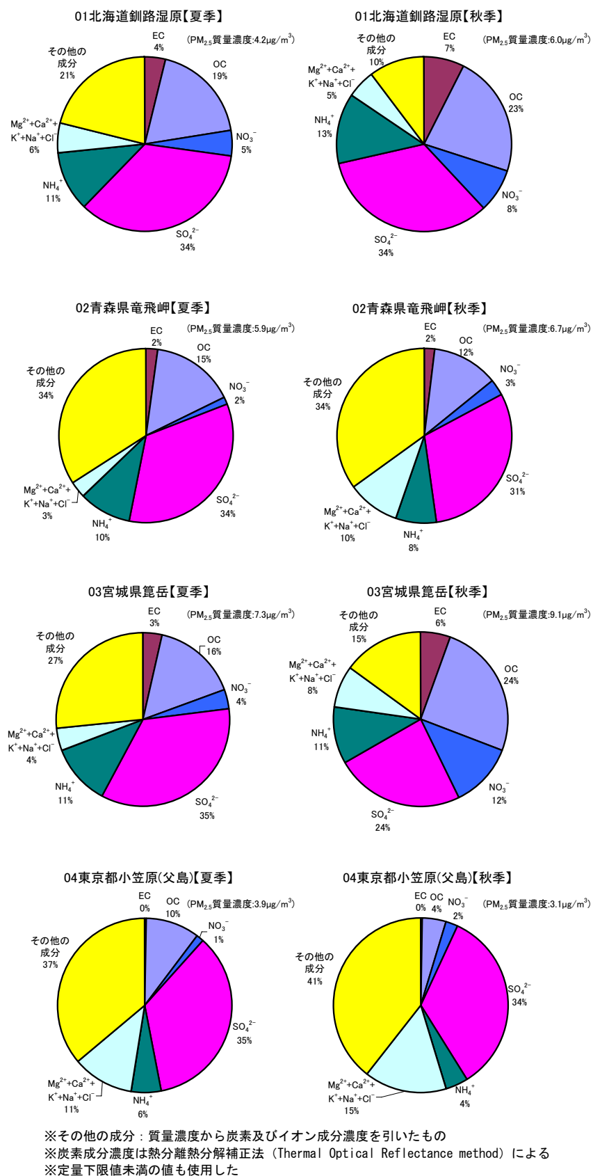
図9(1) PM 2.5 (SASS)炭素・イオン成分等の割合 (平成20年度夏季・秋季の平均値)
