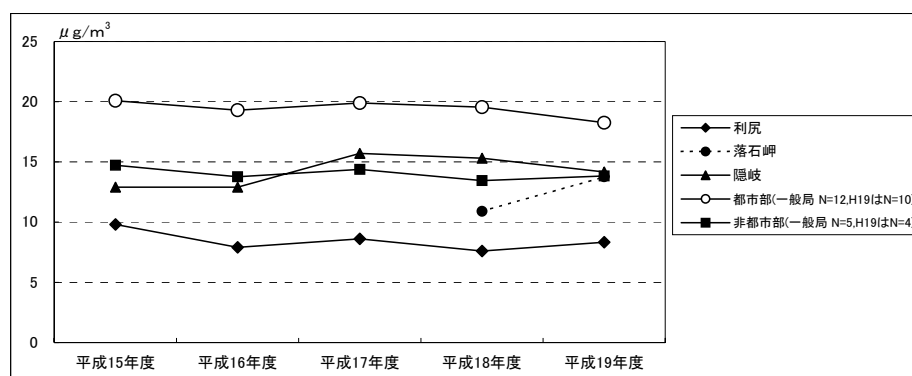
図6 PM 2.5 (50℃加熱式TEOM)質量濃度の年変動 (平成15~19年度：利尻、隠岐、落石岬)
