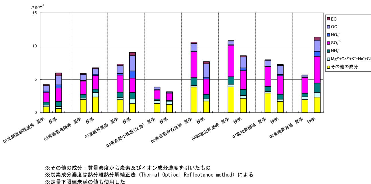
図8 PM 2.5 (SASS)炭素・イオン成分の積み上げ結果 （平成20年度夏季・秋季の平均値）
